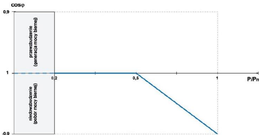
Rys. 5. Charakterystyka sterowania współczynnikiem mocy \cos \varphi w funkcji generowanej mocy czynnej wymagana przez TIEW S.A.
