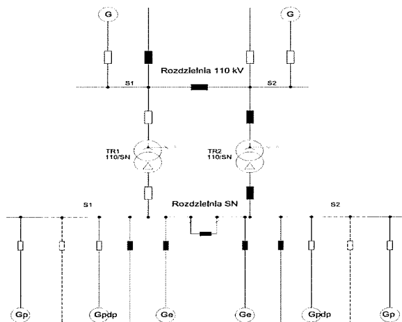
Konfiguracja minimalna stacji 110/SN
