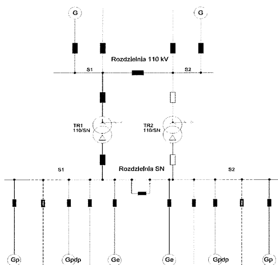
Konfiguracja maksymalna stacji 110/SN
